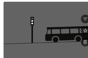
Leeres Info-Profil
